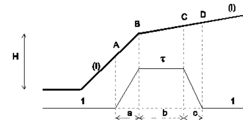
Figure 11 - Points significatifs le long d'un profil topographique schématique pour le calcul du coefficient d'amplification topographique
