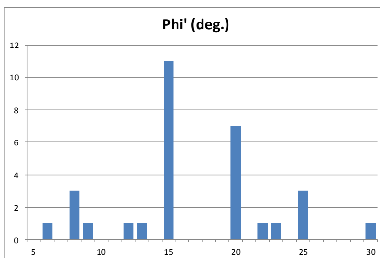
Figure 3 : distribution des valeurs d'angle de frottement calculées par Talren
