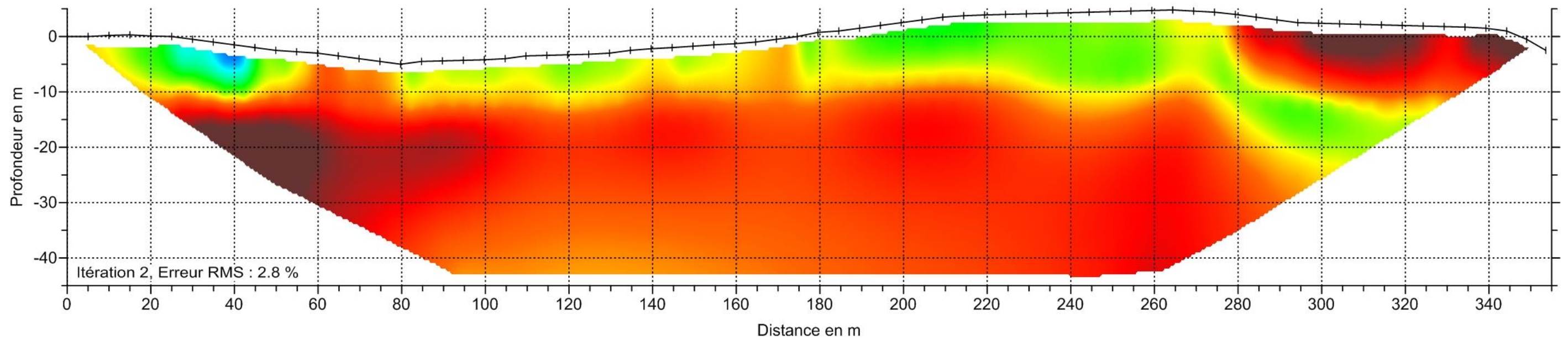
Planche 6 : Résultats du panneau électrique Profil1.
