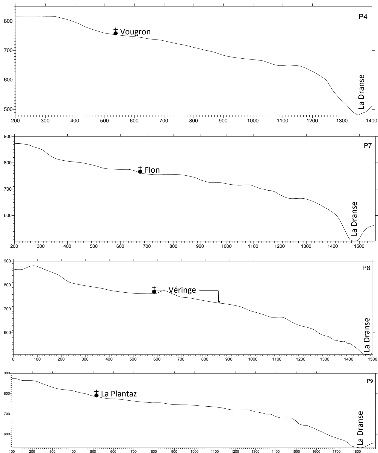
Figure 1 : profils topographiques en travers du versant
