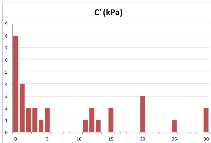
Figure 4 : distribution des valeurs de cohésion calculées par Talren
