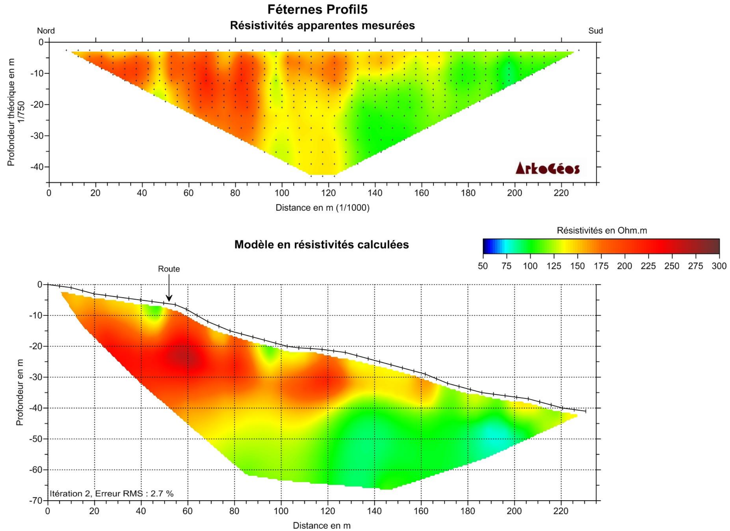
Planche 10 : Résultats du panneau électrique Profil 5.
