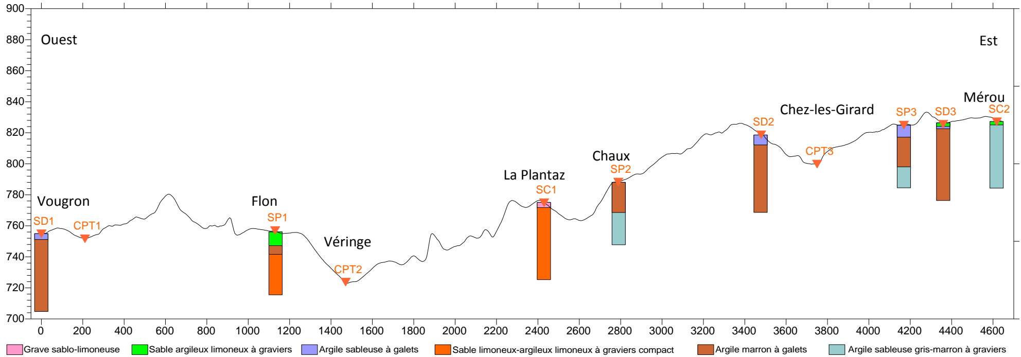
Figure 2 : profil en long ouest-est avec report de la lithologie recoupée par les sondages (échelle verticale dilatée d'un facteur 7.5 par rapport à l'échelle horizontale)
