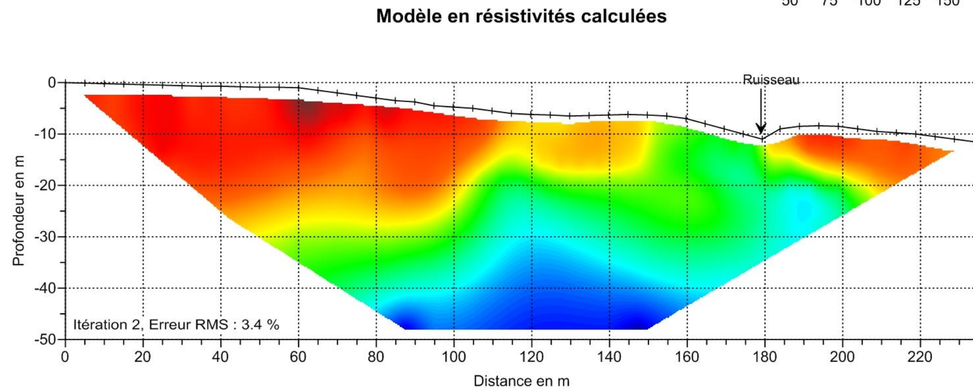
Planche 7 : Résultats du panneau électrique Profil 2.
