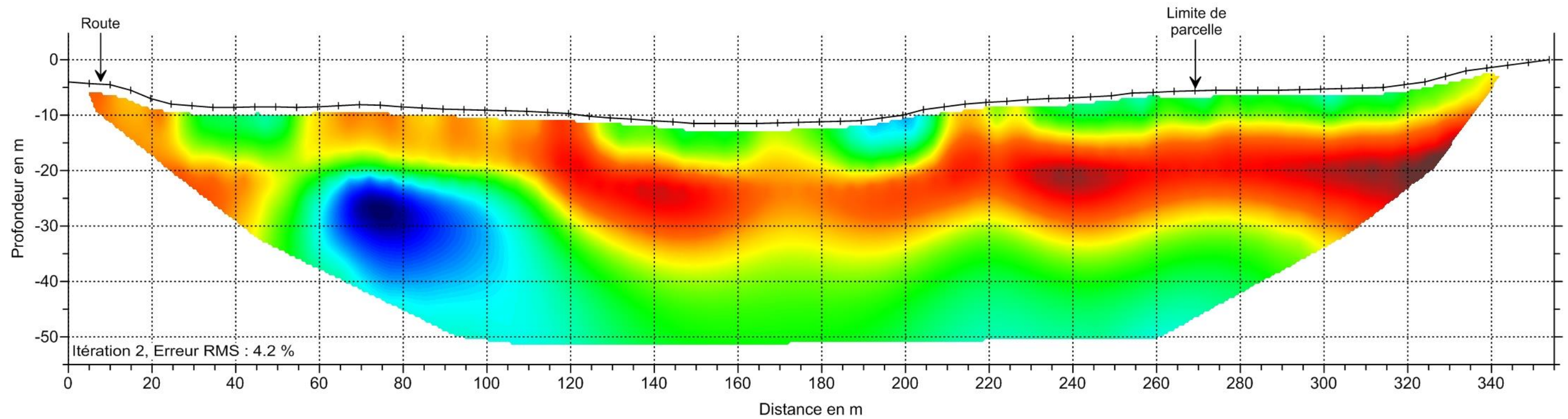
Planche 9 : Résultats du panneau électrique Profil 4.
