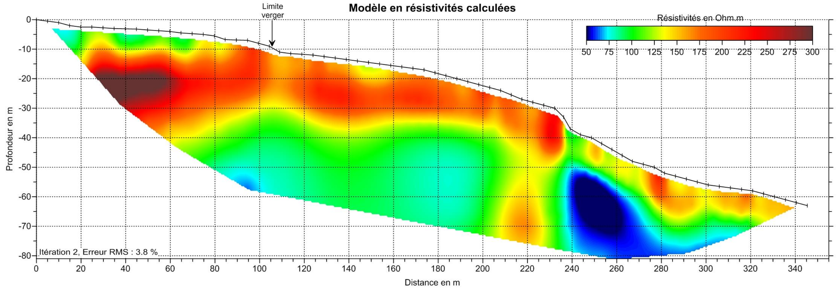
Planche 8 : Résultats du panneau électrique Profil 3.
