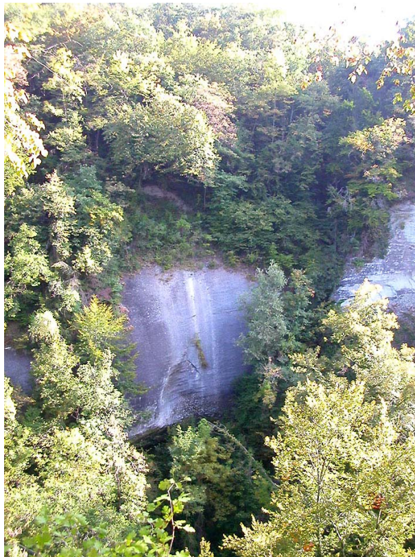
Boussy-ET1 : Gorges du Chéran, au Sud-Est de la commune – Encaissement profond de la rivière.
