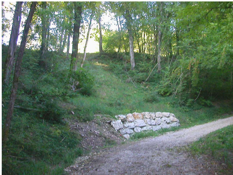
Chainaz-OG1 : Thalweg au Sud des Nants – Confortement de talus par enrochements dans un secteur déstabilisé.
