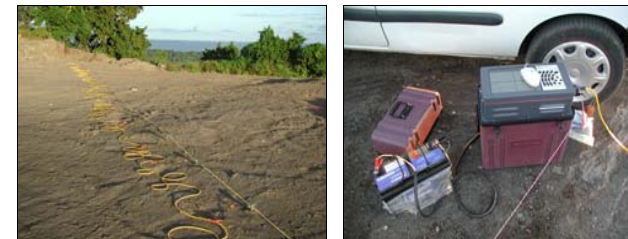
Figure 1 - Dispositif SASW (à gauche : flûte de géophones, à droite : station d'acquisition)
