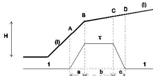
Figure 11 - Points significatifs le long d'un profil topographique schématisé pour le calcul du coefficient d'amplification topographique
