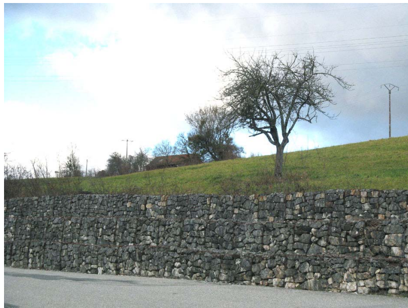
StGermain-OG1 : Carrefour entre le chef lieu et Cernaz – Gabions à étages en confortement de talus.
