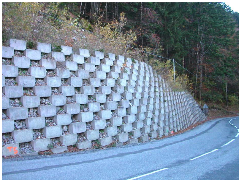
Scionzier-OG2 : RD4, sous la Pététaz – Confortement de talus par éléments assemblés.
