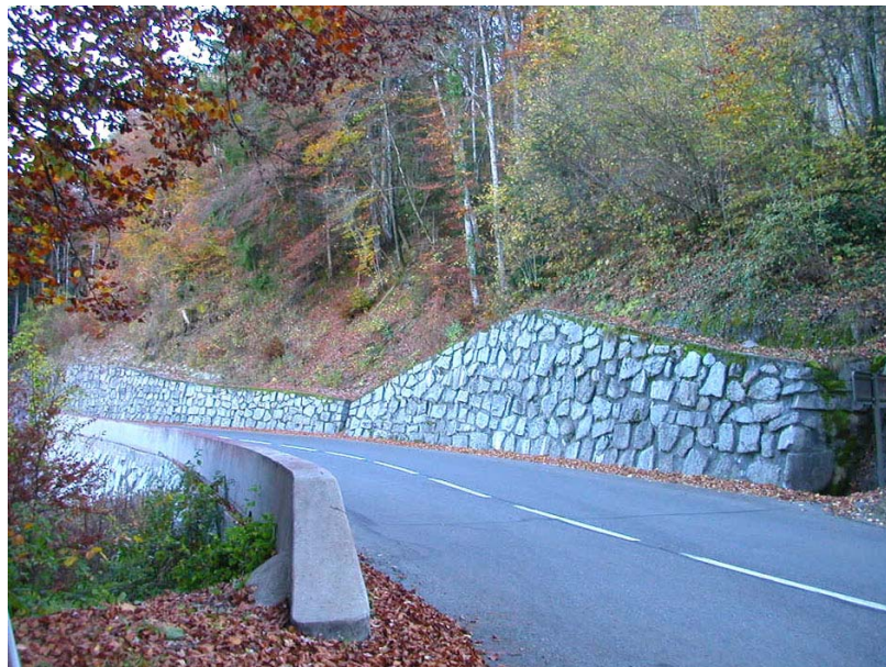
Scionzier-OG3 : RD4, sous le hameau de Neyrolles – Confortement de talus par des murs en pierres maçonnées.
