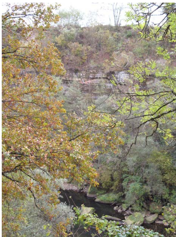
Sales-EP1 : Rive gauche du Fier, à l'Ouest de Chez Perret – Gorges délimitées par des parois de molasse de plus de 20-30m de haut.
