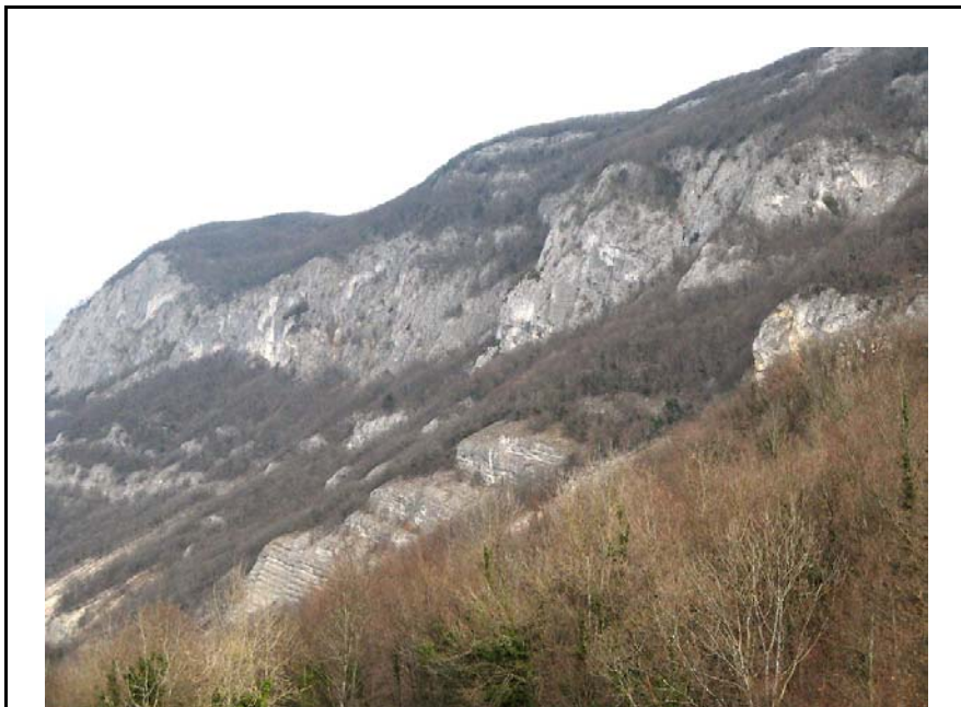
Clarafond-EP3 : Au dessus de la RD908a menant d'Arcine à Entremont – Vue générale sur les falaises qui dominent le versant.
